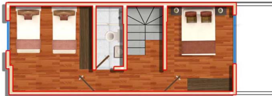
PLANTA ALTA
